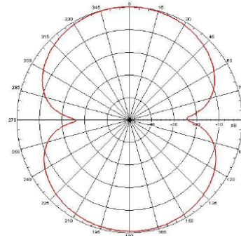
E-PLANE
