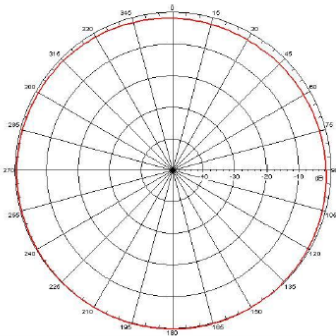
H-PLANE
